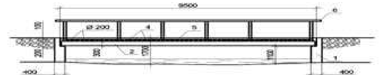
Манбаъ: Кўпруки Помир, нақшаи кўпруки № 80, андозаҳои намунавӣ
